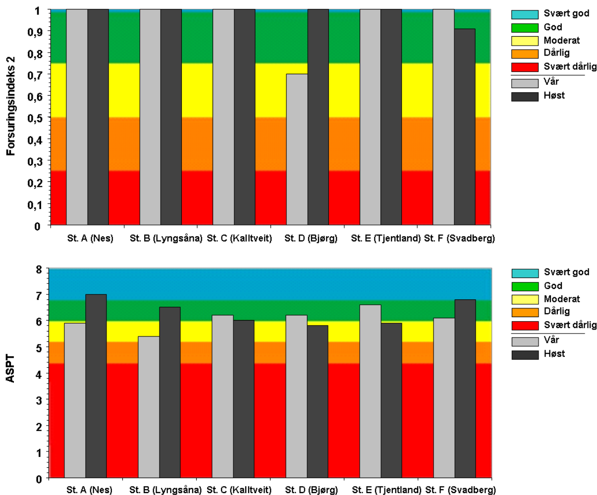
Figur 4: Forsuringssindeks 2 (øverst) og ASPT-indeks (nederst) for bunndyrstasjoner i Årdalsvassdraget vår (05.06) og høst (28.10) 2011.
