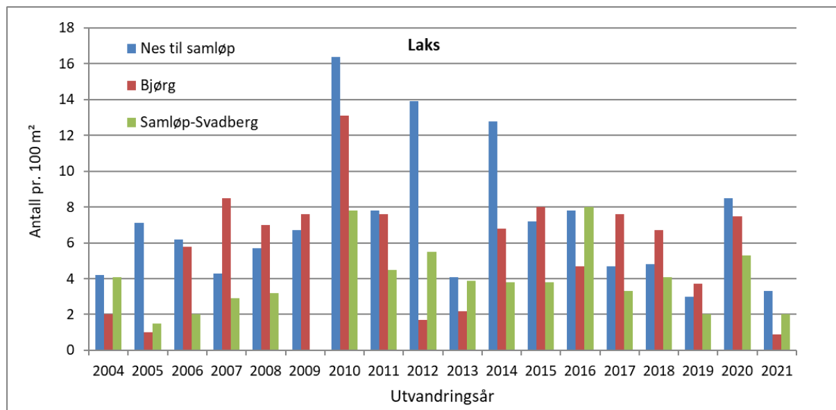
Figur 4.11. Presmoltetthet av laks i elveavsnittene "Nes til samløp", "Bjørg" og "Samløp til Svadberg" fra 2004-2020. Tidspunkt oppgitt som utvandringsår for smolt, som vil si at presmolt fisket november/desember 2020 vil vandre ut som smolt i 2021.
