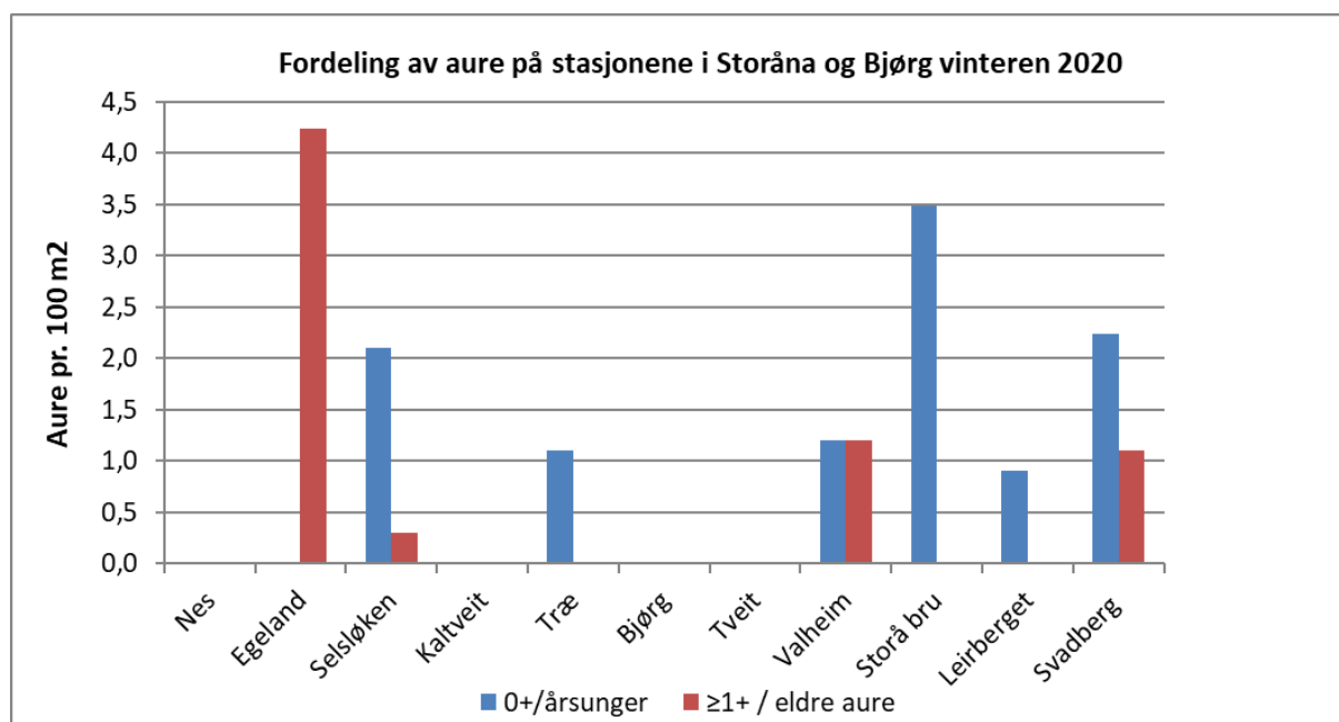
Figur 4.7. Tetthet av aure pr 100 m 2 på de ulike stasjonene elfisket i Storåna og Bjørg november/desember 2020.
