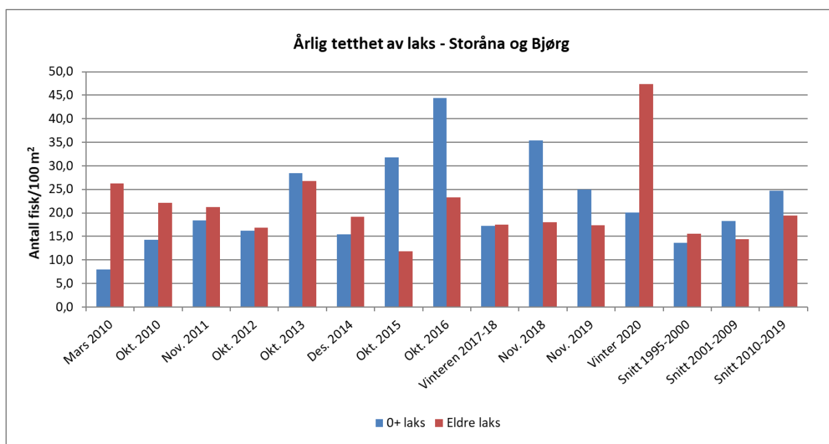
Figur 4.3. Tetthet av laksunger i Storåna og Bjørg fra 2000 til november/desember 2020. Merk at fisket er utført til ulike tider av året. Tetthetene fram til og med 2009 er basert på fiske på 6 stasjoner. Fra 2010 inkluderer undersøkelsene 11 stasjoner. Gjennomsnitt for alle undersøkelser for periodene 1995-2000, 2001-2009 og 2010-2019, da antall stasjoner ble utvidet, er også vist.
