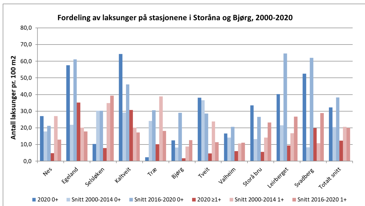
Figur 4.5. Tetthet av laksunger pr. 100 m 2 på de enkelte stasjonene i Storåna og Bjørg, sammenlignet med gjennomsnittsverdier for tetthet før og etter minstevannføring ble innført i 2015.
